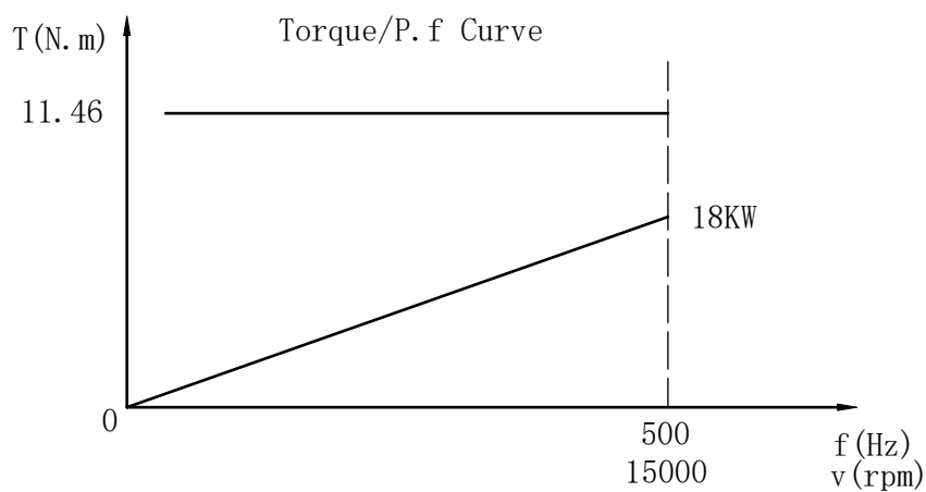
扭矩/功率曲线
